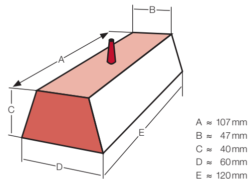
Fig. 33: Test box
